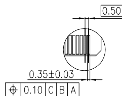
DETAIL:C SCALE 2:1
