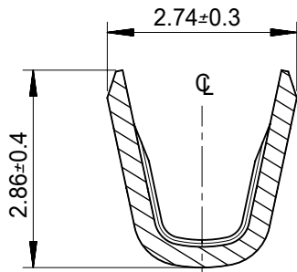
SECTION A-A Scale 10:1
