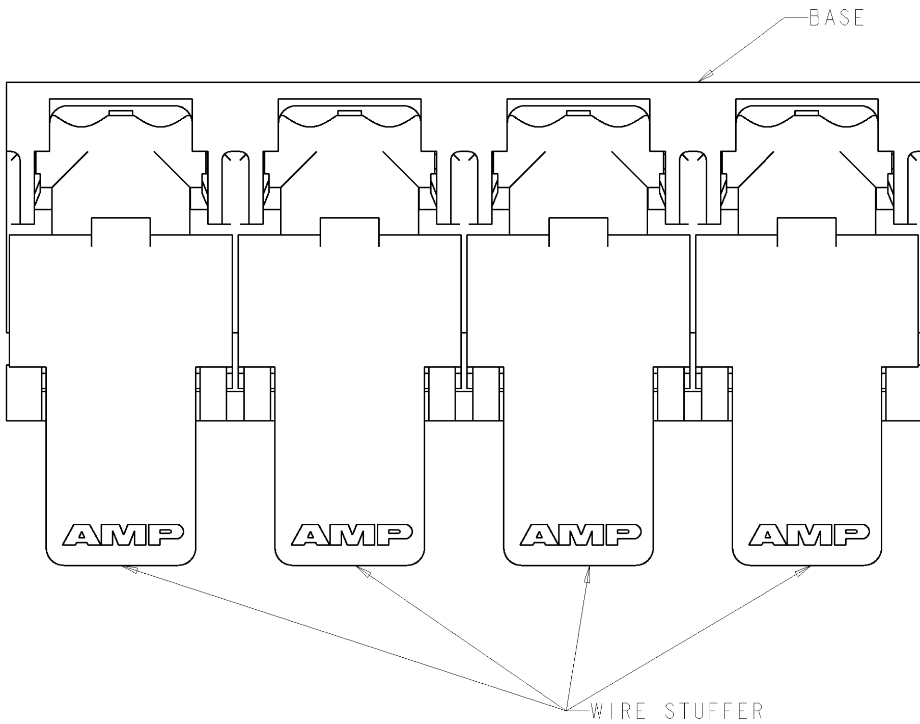
1339376-1 SHOWN SCALE 4:1
