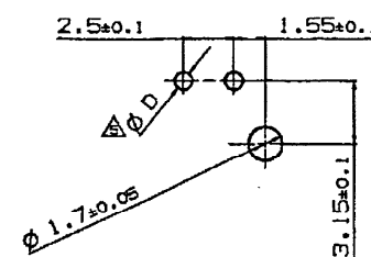
取付基板寸法 FIG. 1
