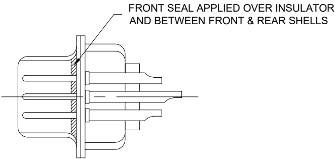
DETAIL A-A
