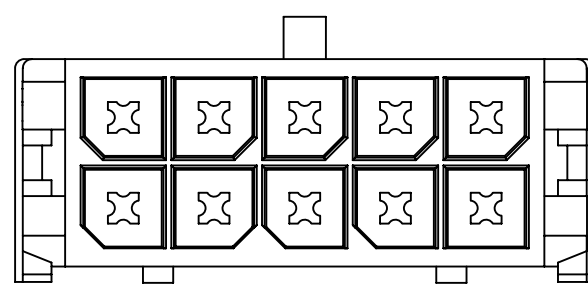
10CKT
