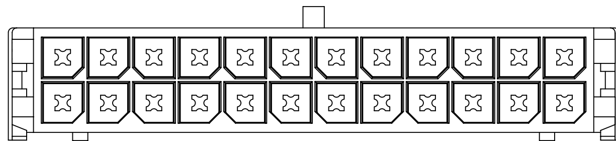
12CKT
