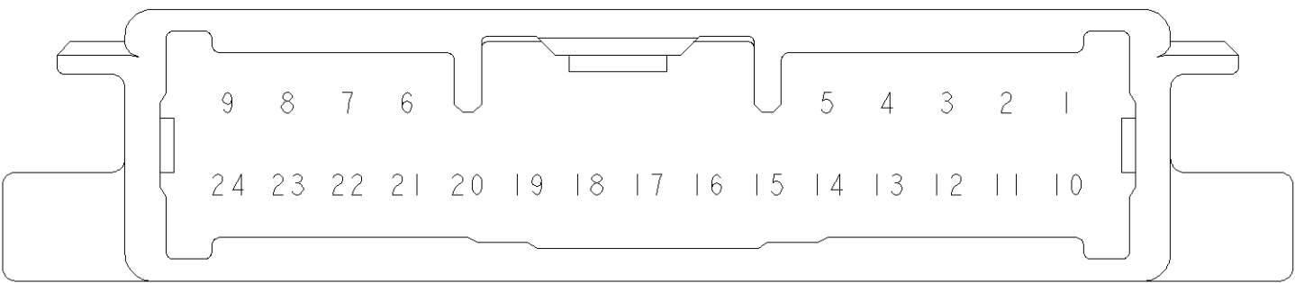
△ FIG.1 CONTACT COMPOSITION コンタクト回路構成
