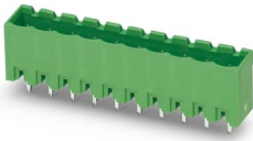
图为10位穿墙式连接器
