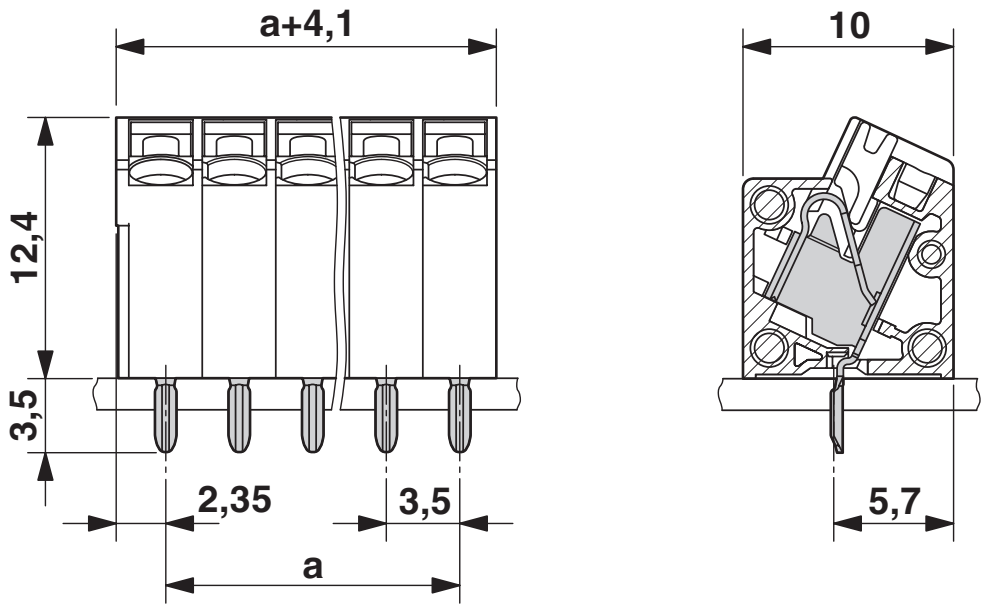
尺寸图
