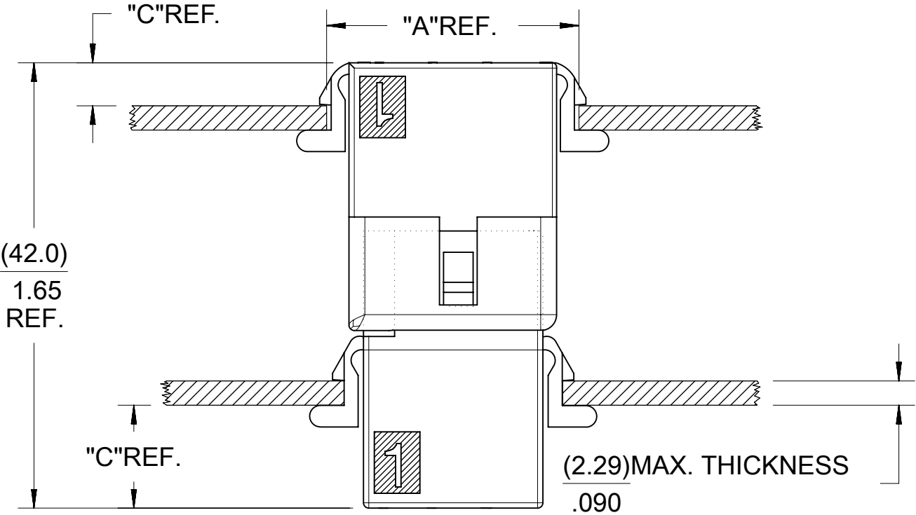
RECEPTACLE 1292-R
