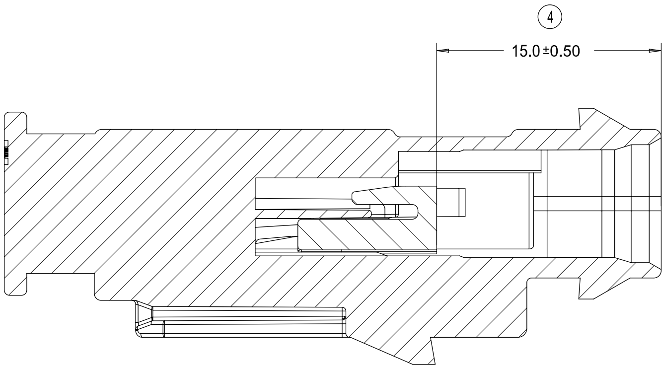
SECTION V-V
