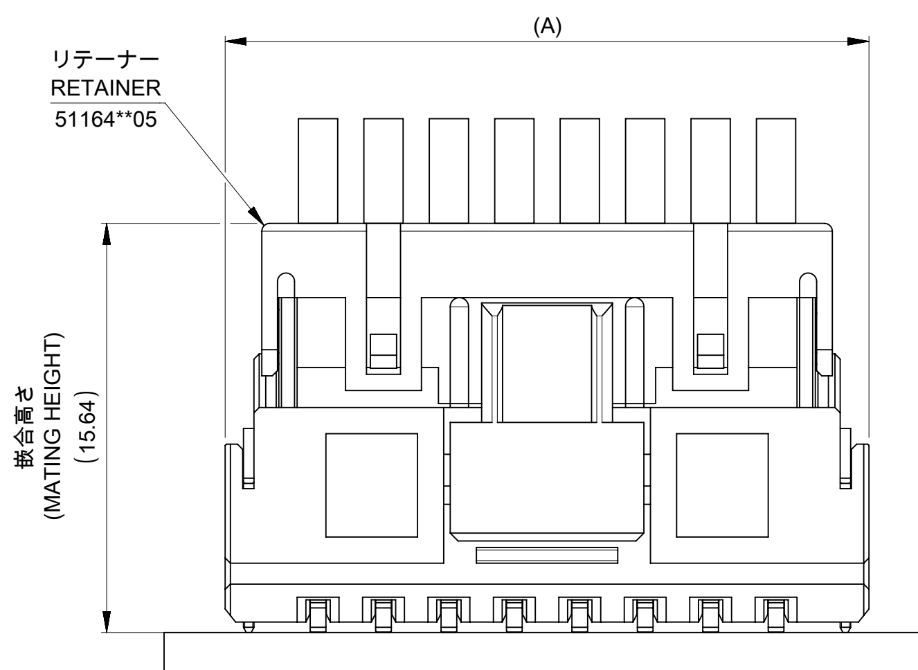
嵌合狀態圖 MATED CONNECTORS
