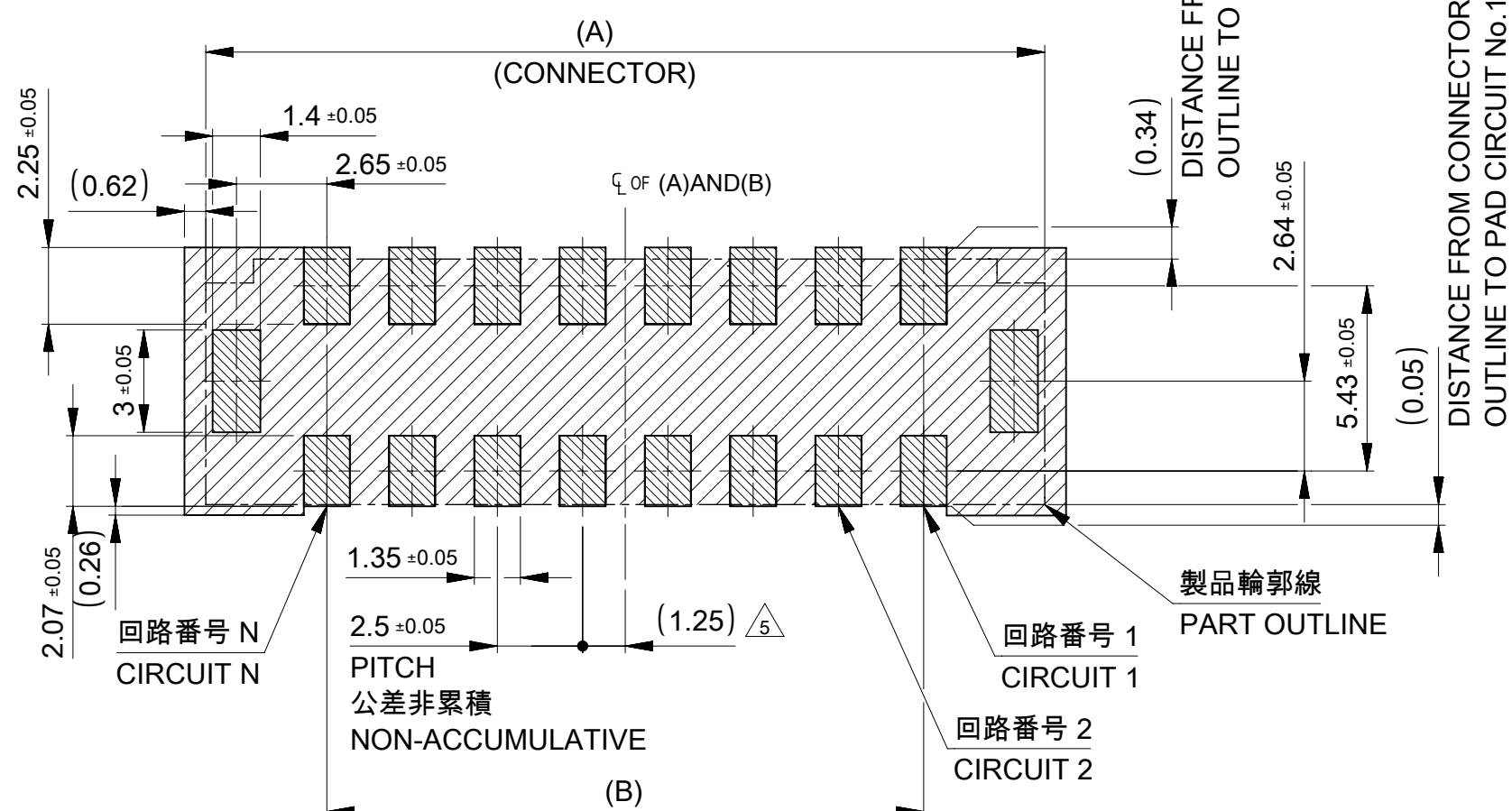
製品レイアウト PRODUCT LAYOUT
