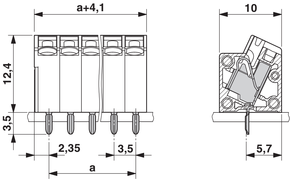
尺寸图
