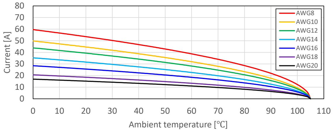
D5300 3P GOLD or PdNi &amp; Gold flash
