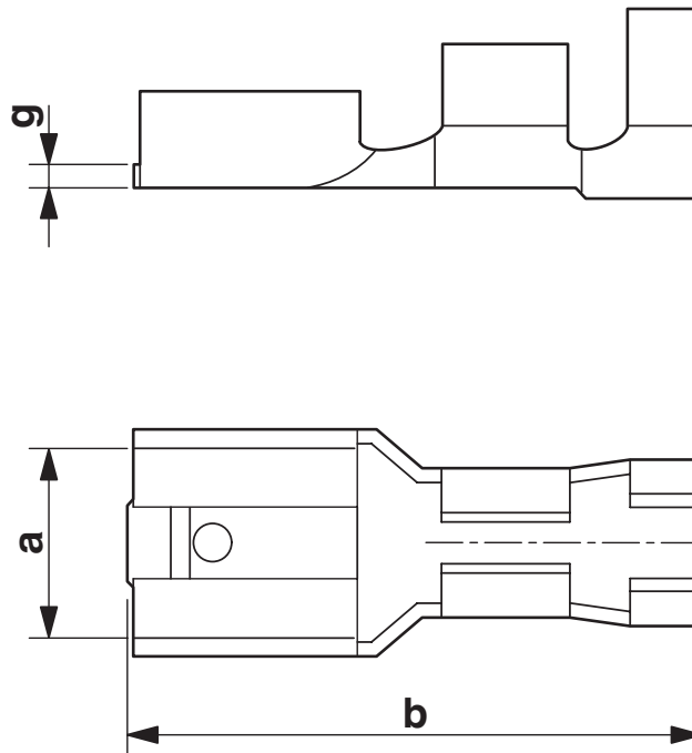
尺寸图
