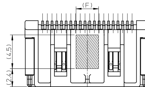
吸着範囲 VACUME AREA
