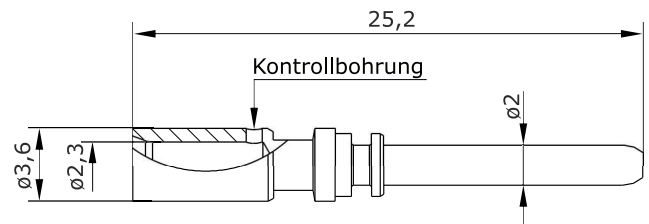
Hauptabmessungen Kontaktstift
