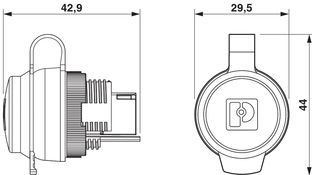
尺寸图
