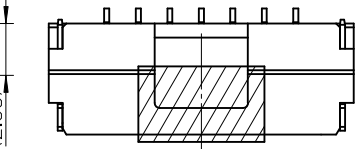
カプトンテープ付き WITH KAPTON TAPE
