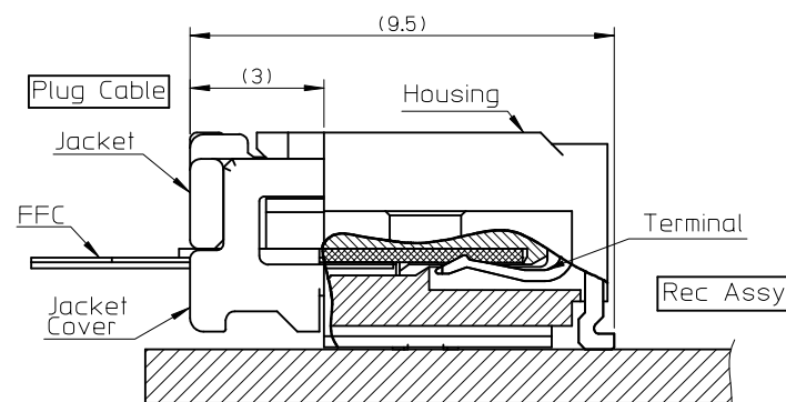
嵌合断面図
