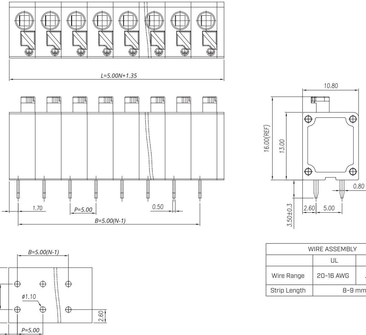
P.C.B. LAYOUT
