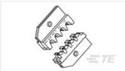
TE Part #539773-2 DIE FUER MINI MIC
