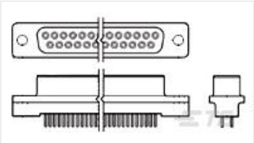
TE Part #5745078-4 HD-20 RCPT 25P VERT FFSCRLK
