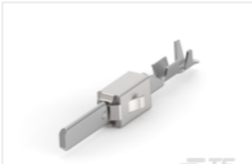
TE Part #5-963860-1 TAB 2.8x0.8 CONTACT CS SRC Sn
