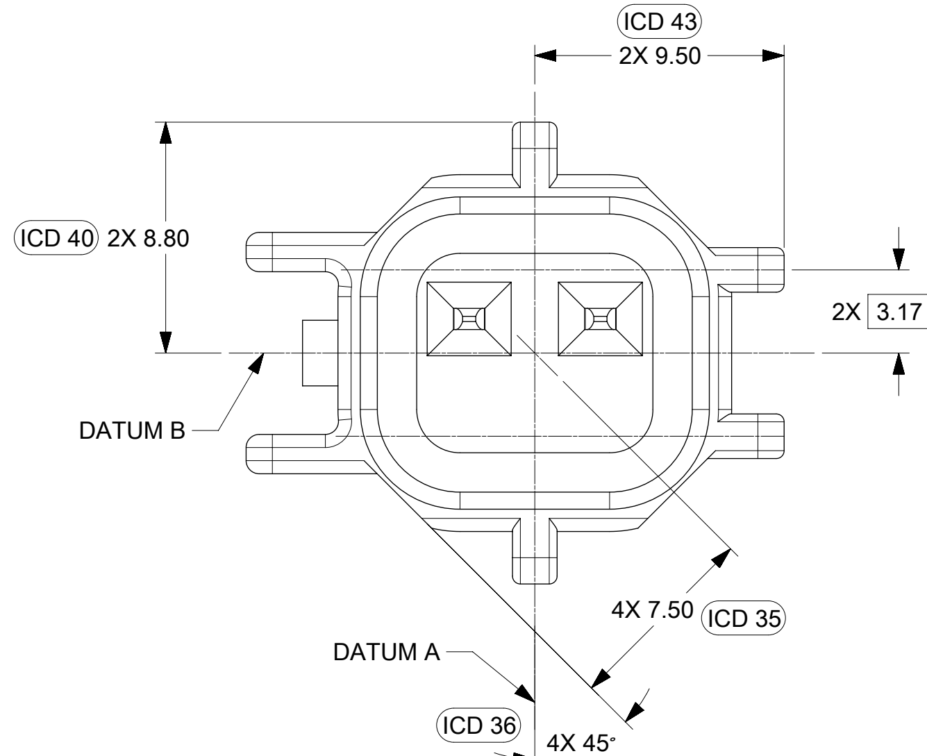
OPTION E
