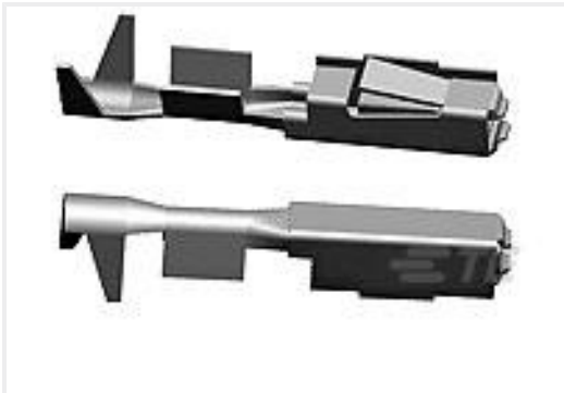
TE Part #5-928999-5 MQS0,63 Au rec LL unseal. >0,2-0,35
