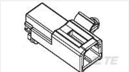
TE Part #178602-1 070 MULTILOC CAP HSG PANEL LOC
