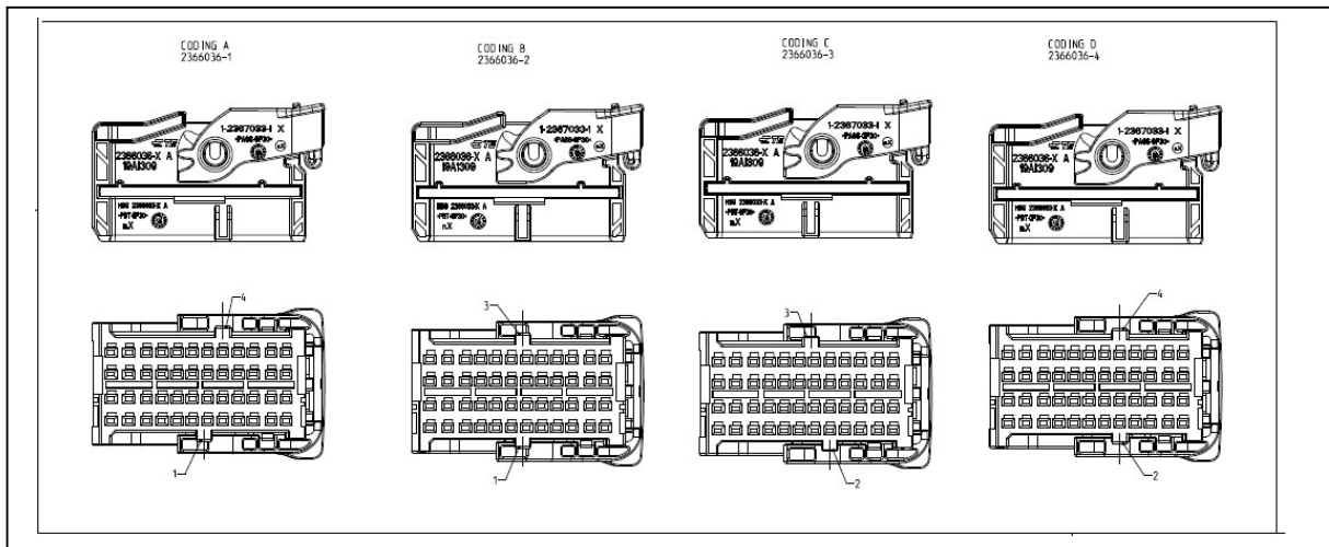
Figure 2.1.3 Four Coding of Plug Connector 图 2.1.3 母端连接器的 4 个 Coding
