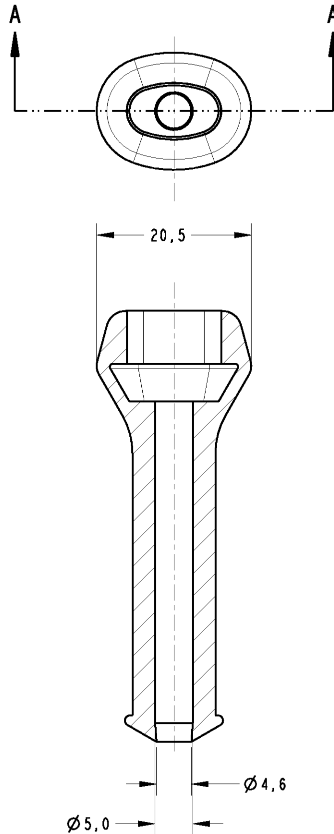
SECTION A-A
