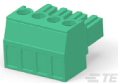
TE Part # 284507-4 4 POS TERMI-BLOK PLUG STAC 3,8
