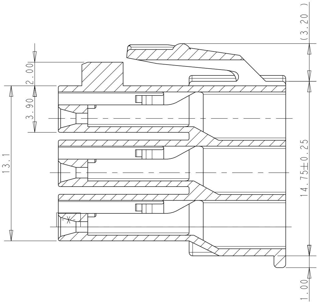
SECTION A-A
