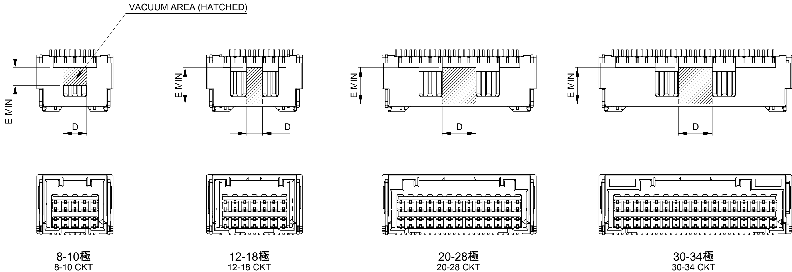
極数別ハウジング形状および吸着エリア HOUSING SHAPE AND VACUUM AREA AT EACH CKTS
