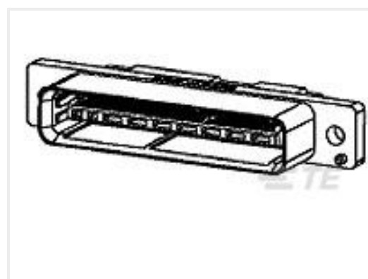
TE Part #6-292233-0 1.5 MINI CT DRAWER 60P PLUG
