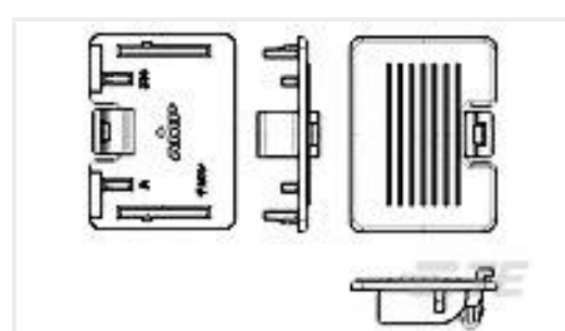
TE Part #1-1123919-4 1.5 MINI CT DUST COVER
