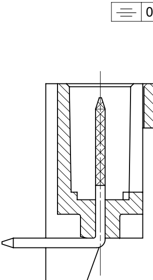
SECTION L-
