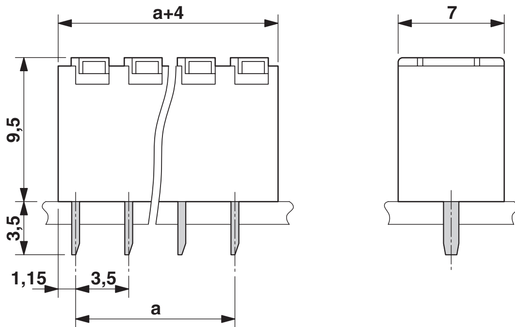
尺寸图
