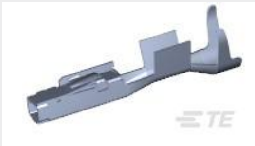
TE Part #7-1452671-2 MCON 1.2 LL REC SWS AU
