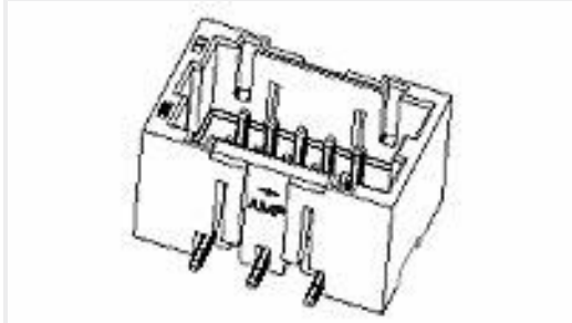
TE Part # 3-292229-0 1.5 MINI CT D/R SMT 30P V ONTA
