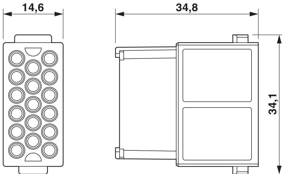
尺寸图
