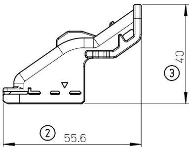
LONG TYPE 560189-0111
