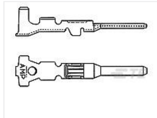
TE Part #282109-1 MINI MIC TAB CONTACT
