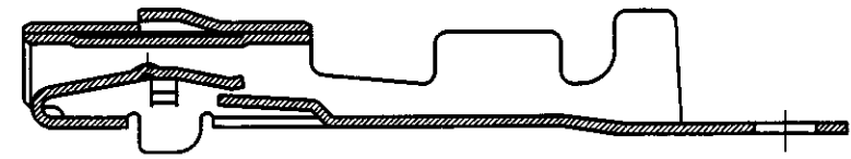
断面 A-A (SECT. A-A)
