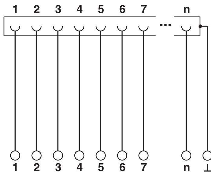
电路图
