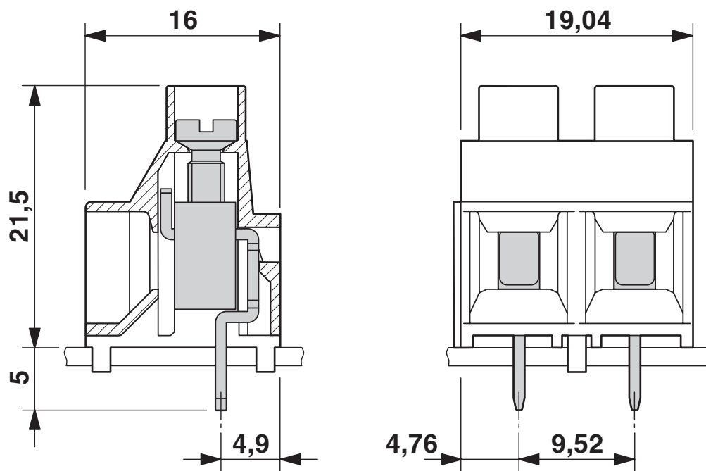
尺寸图
