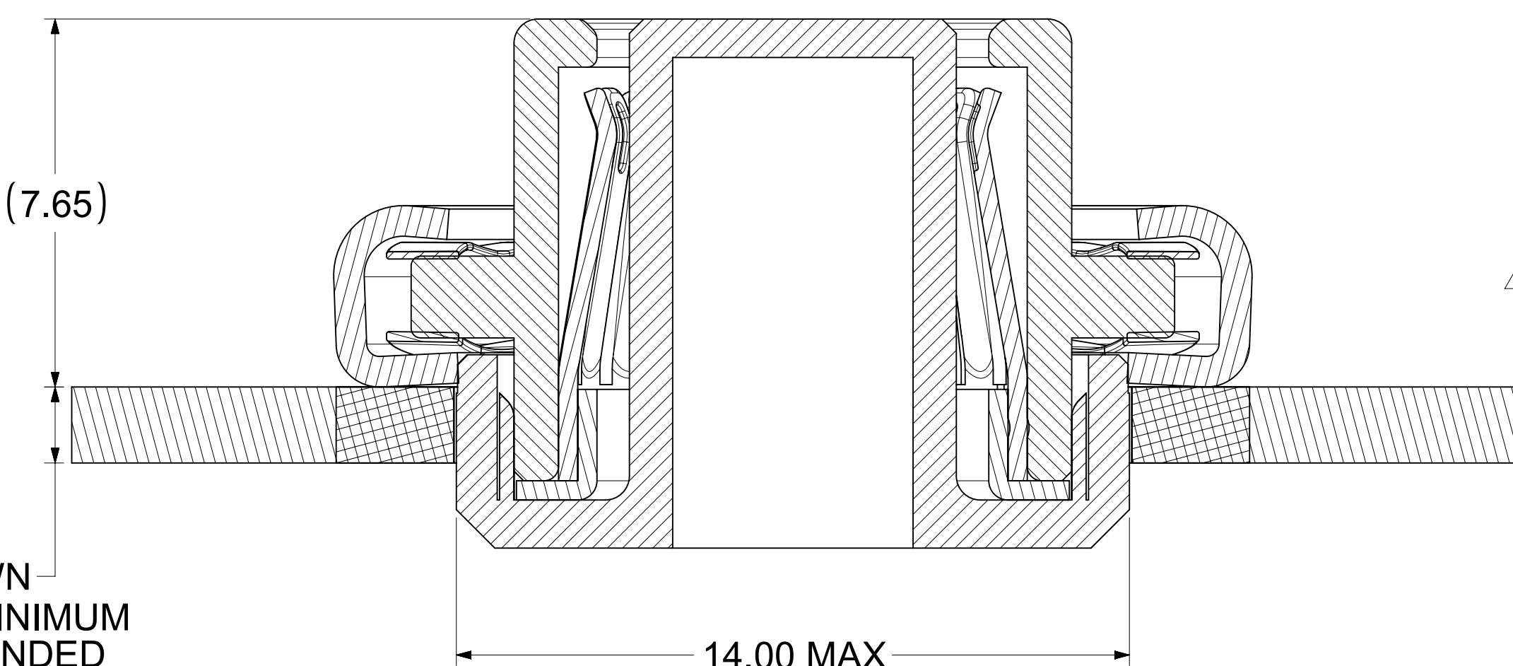
SECTION A-A
