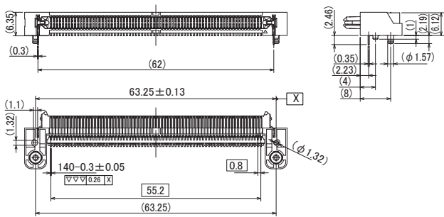
ER8L-140P-0.8SH(##)
