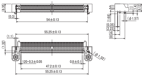
ER8-120P-0.8SH(##)
