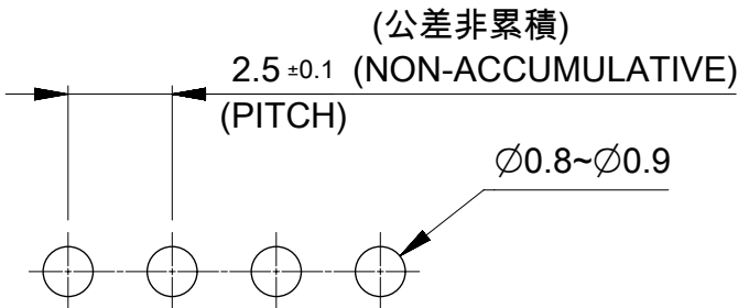
基板取付穴推奨寸法 RECOMMENDED PCB HOLE DIMENSION (t=1.6)
