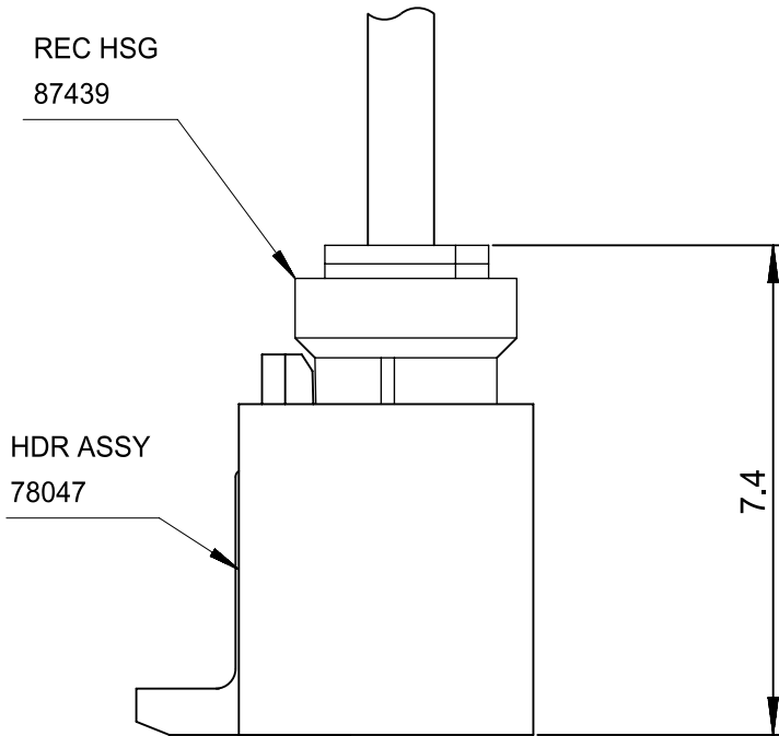
嵌合状態図 MATED CONNECTORS
