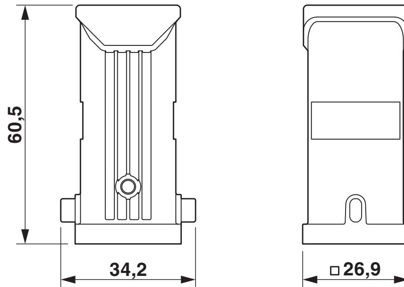
尺寸图
