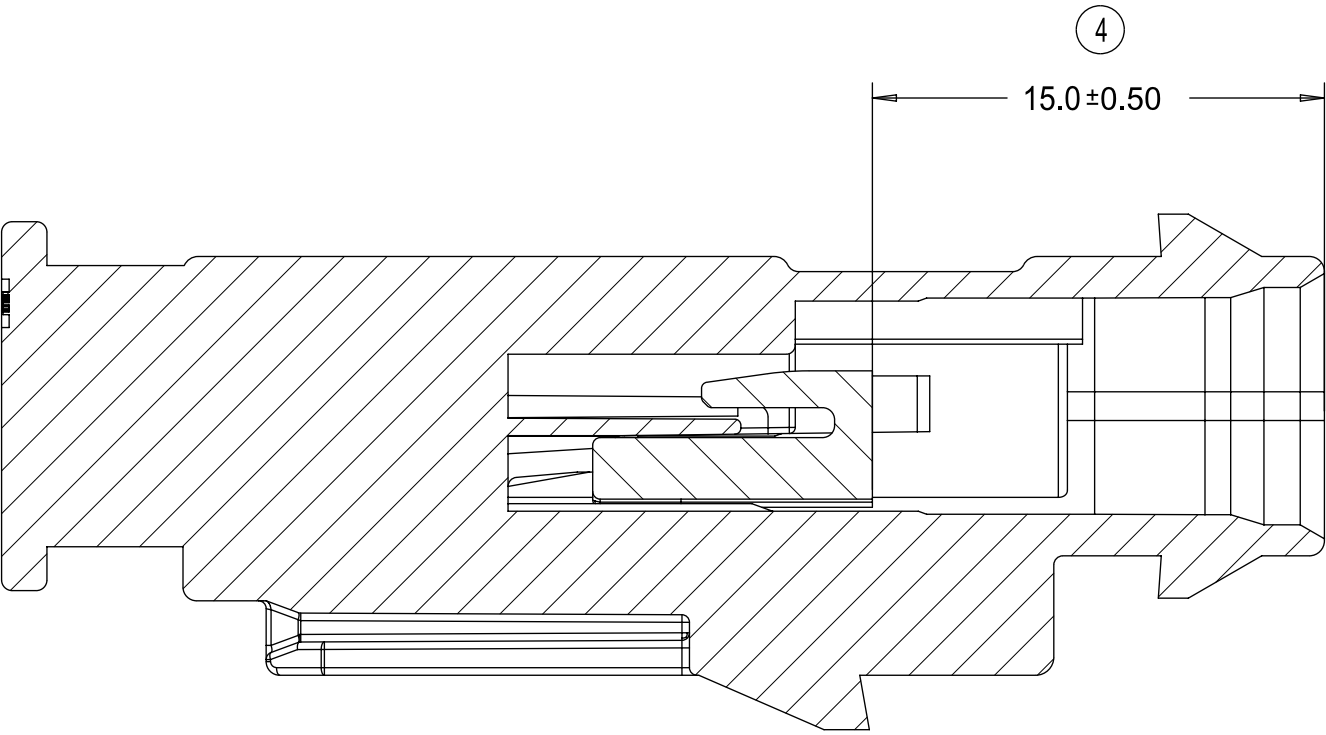
SECTION V-V
