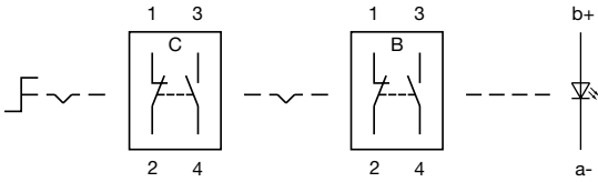
Wiring diagram 288
