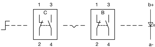
Wiring diagram 285
